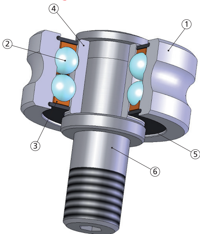
cuscinetto/bearing
