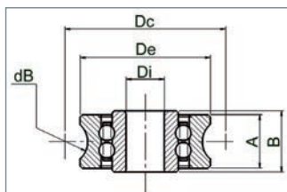
cuscinetto/bearing
